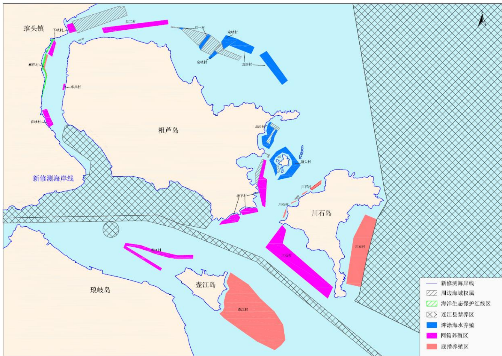
图 1.4-1 项目用海总平面布置图
