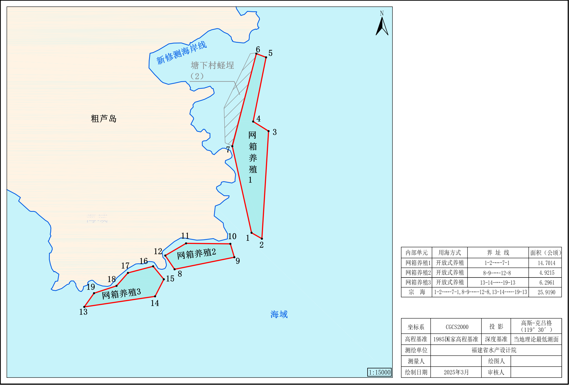
连江县琯头镇海水养殖项目(塘下村海水养殖区)宗海界址图
