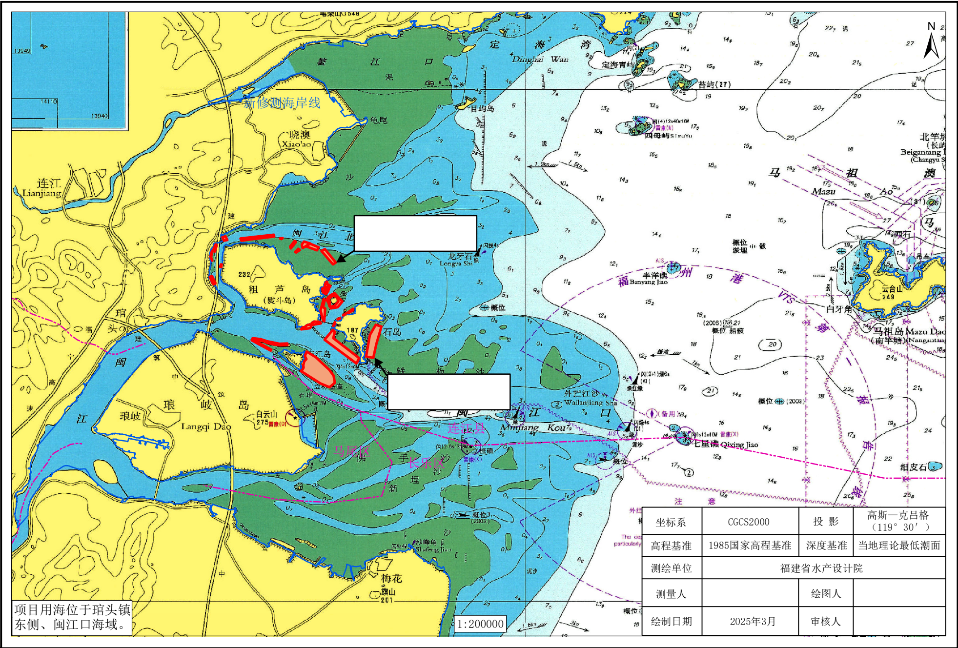
连江县琯头镇海水养殖项目宗海位置图
