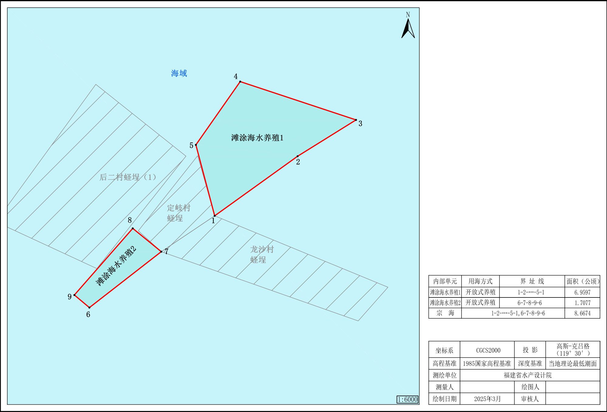
连江县琯头镇海水养殖项目(定岐村海水养殖区)宗海界址图
