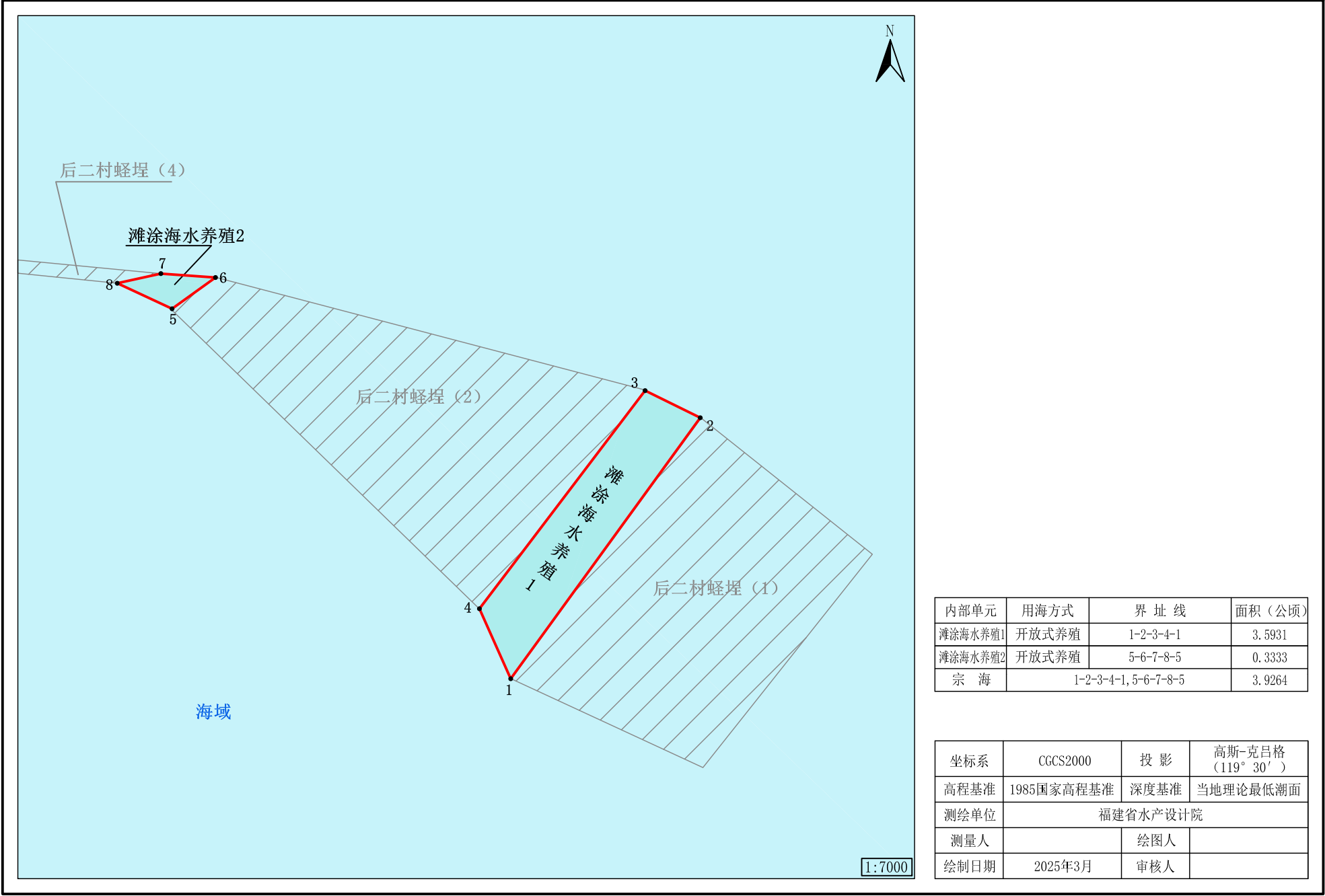
连江县琯头镇海水养殖项目(后一村海水养殖区)宗海界址图
