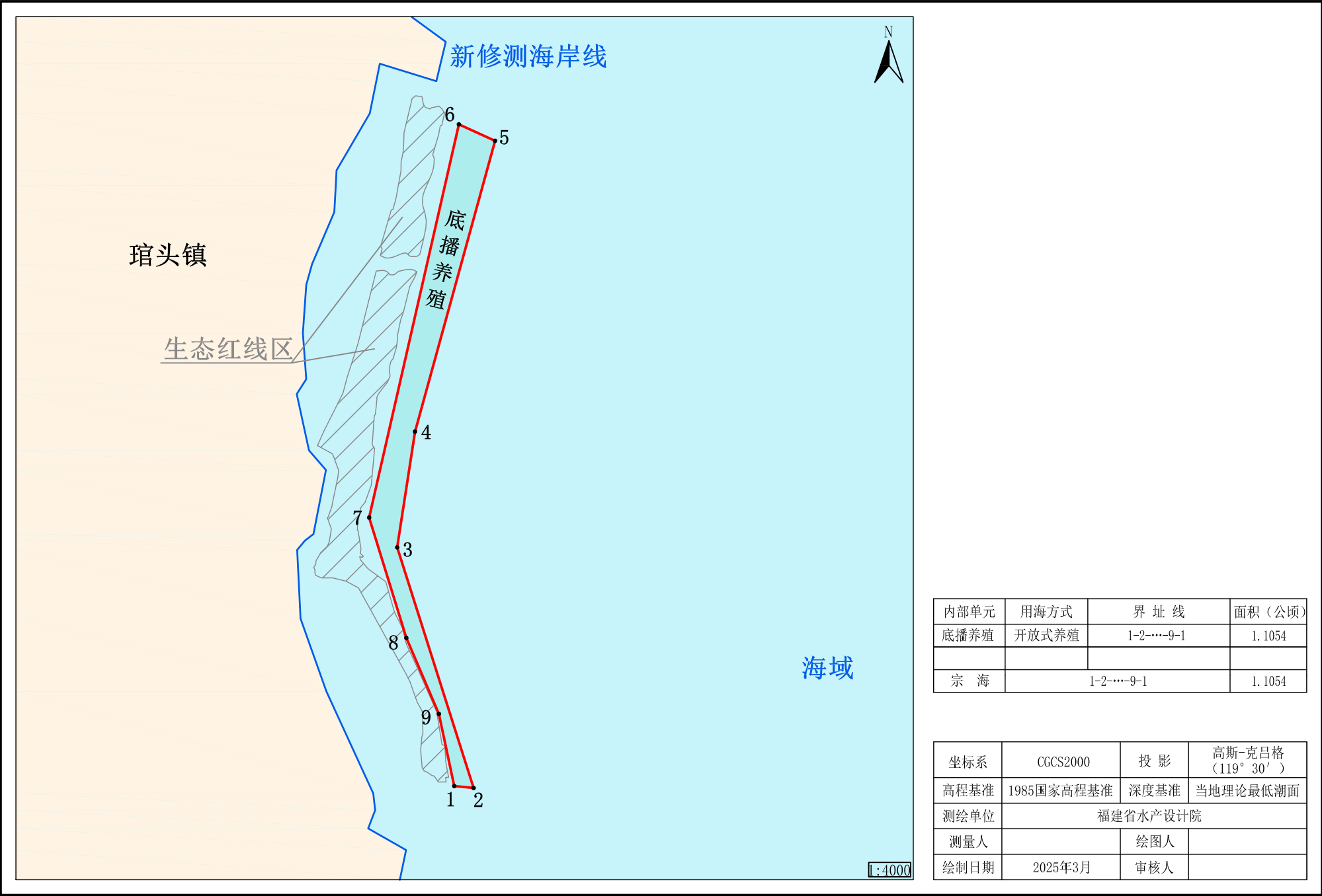
连江县琯头镇海水养殖项目(寨洋村海水养殖区)宗海界址图
