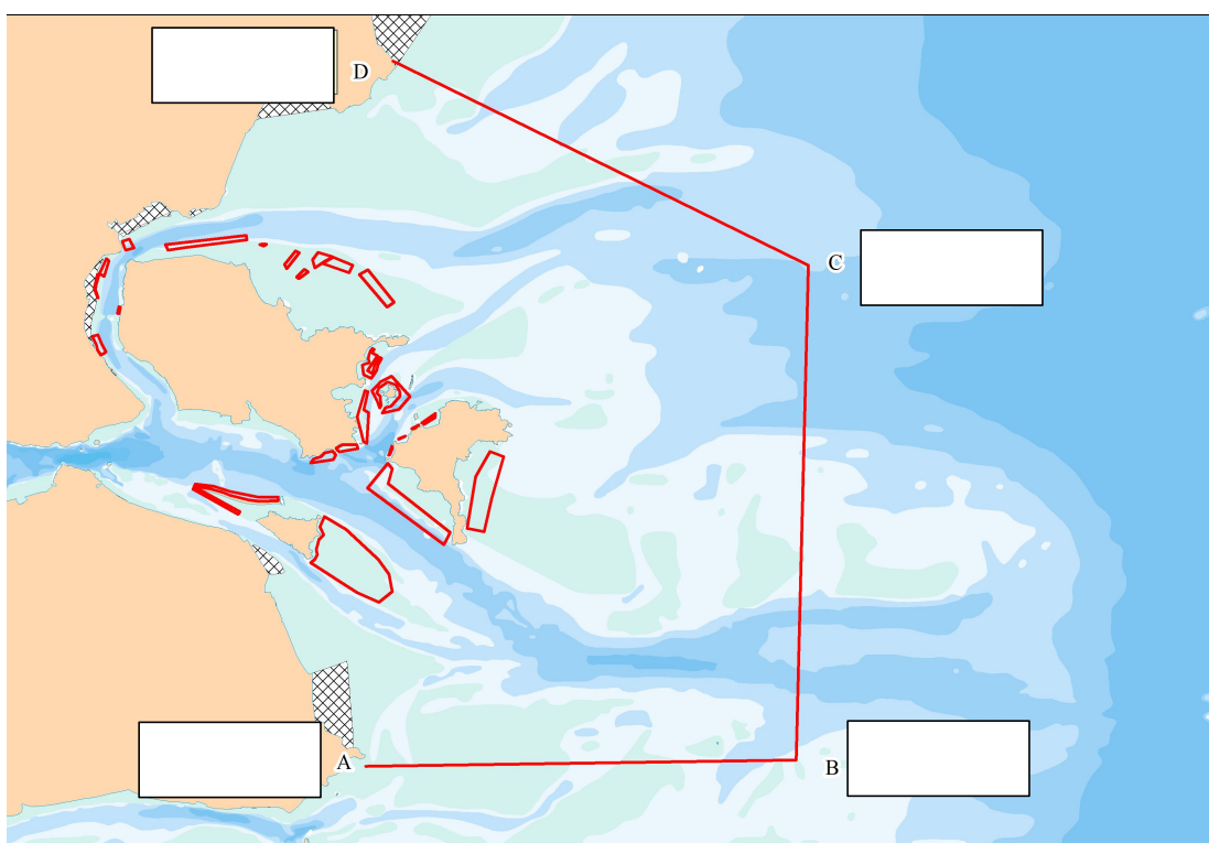
图 1.6-1 本项目用海论证范围图
