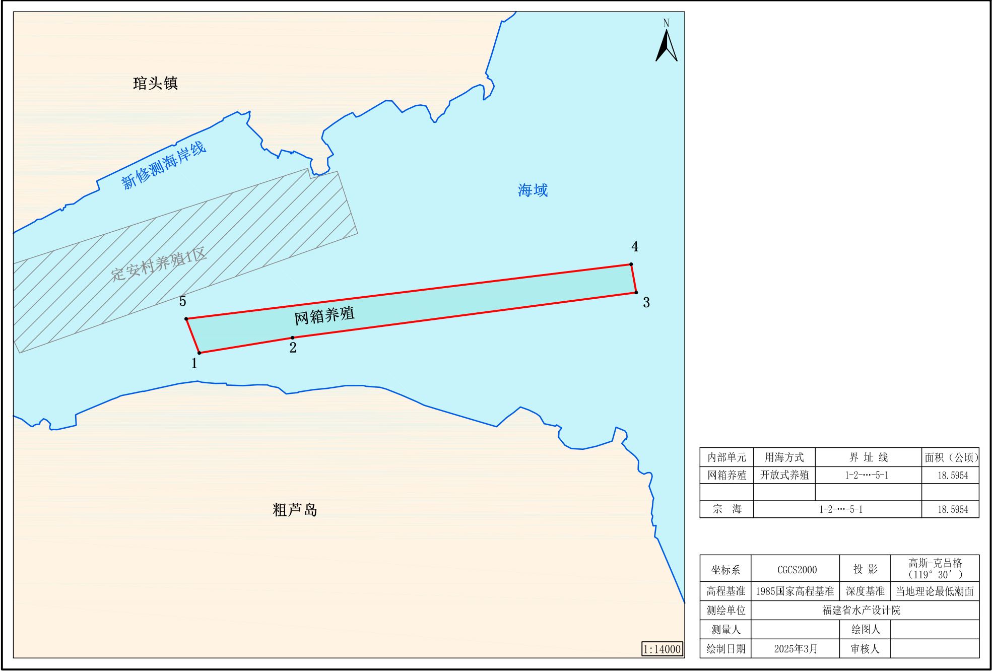
连江县琯头镇海水养殖项目(后二村海水养殖区)宗海界址图
