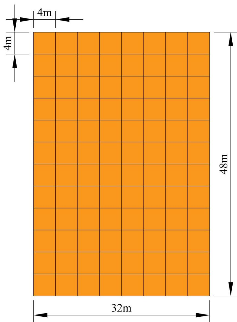
图 1.4-2 网箱养殖基本单元平面示意图
